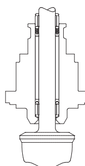
Engaxetamento Padrão p/ Vácuo c/ Anéis "V"
