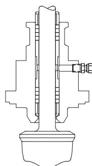
Engaxetamento Duplo c/ Anéis Quadrados e Conexão para Lubrificador
