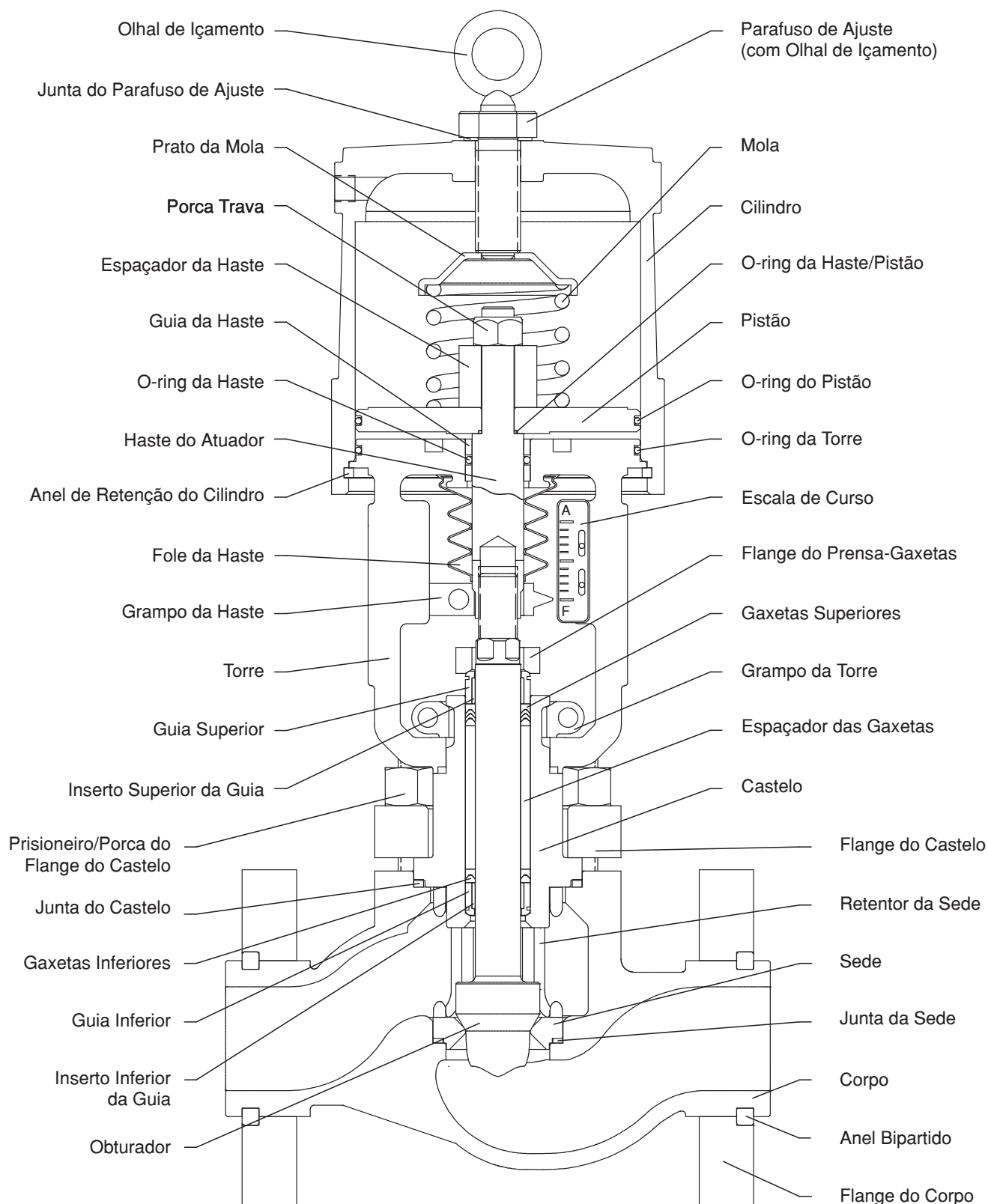
Figura 2 - Válvula de controle GL̄
