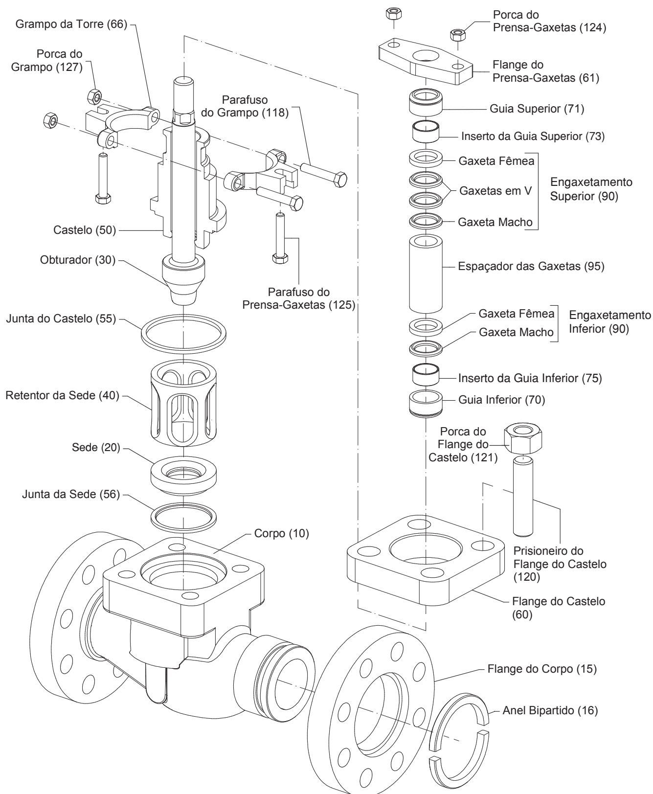
Figura 3 - Vista Explodida do Subconjunto do Corpo
