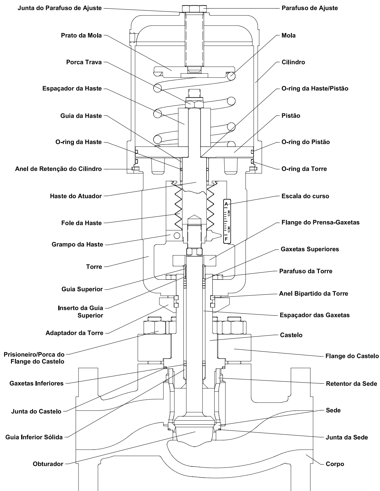
Figura 2 - Válvula de controle GLI
