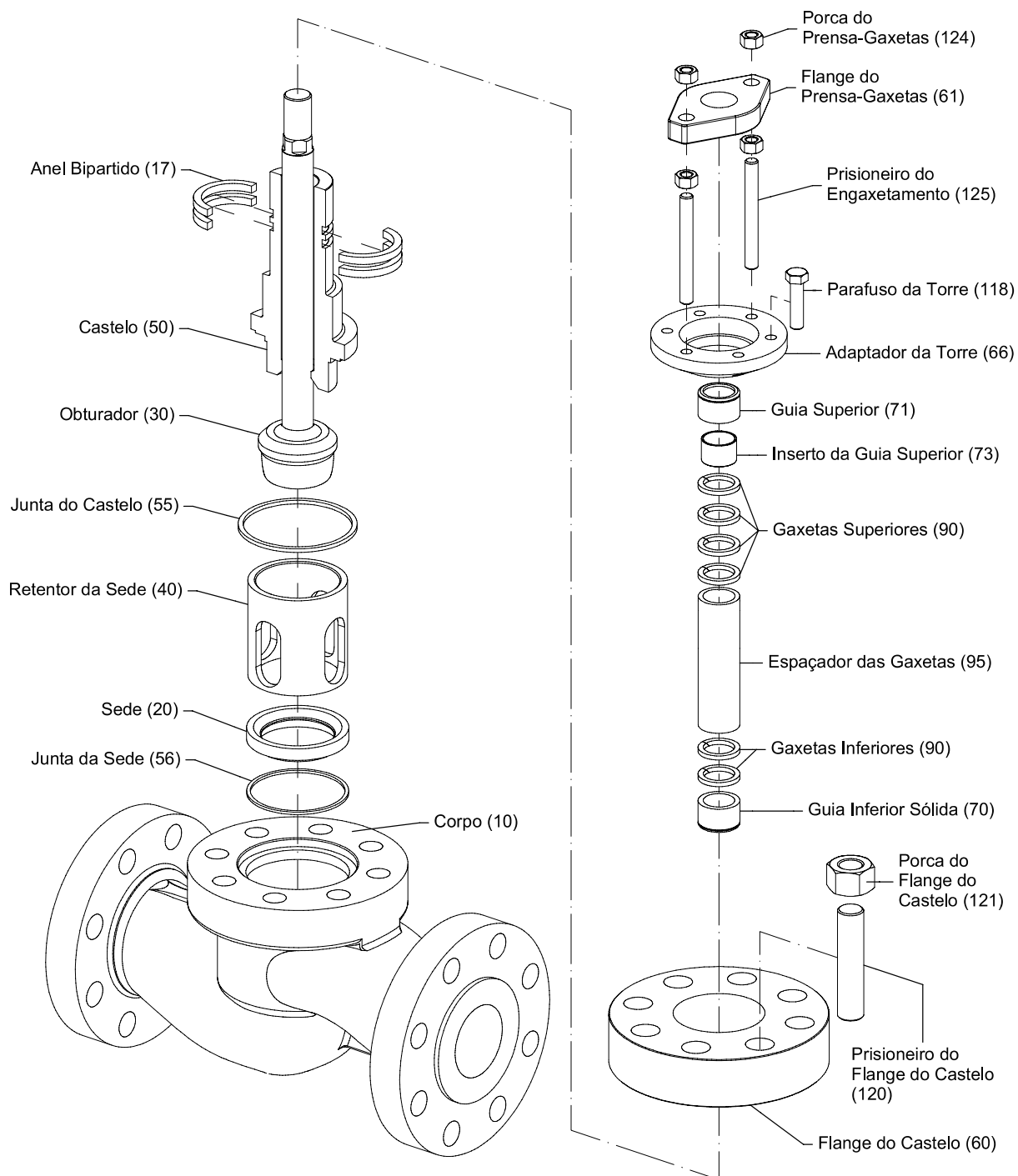
Figura 3 - Vista Explodida do Subconjunto do Corpo
