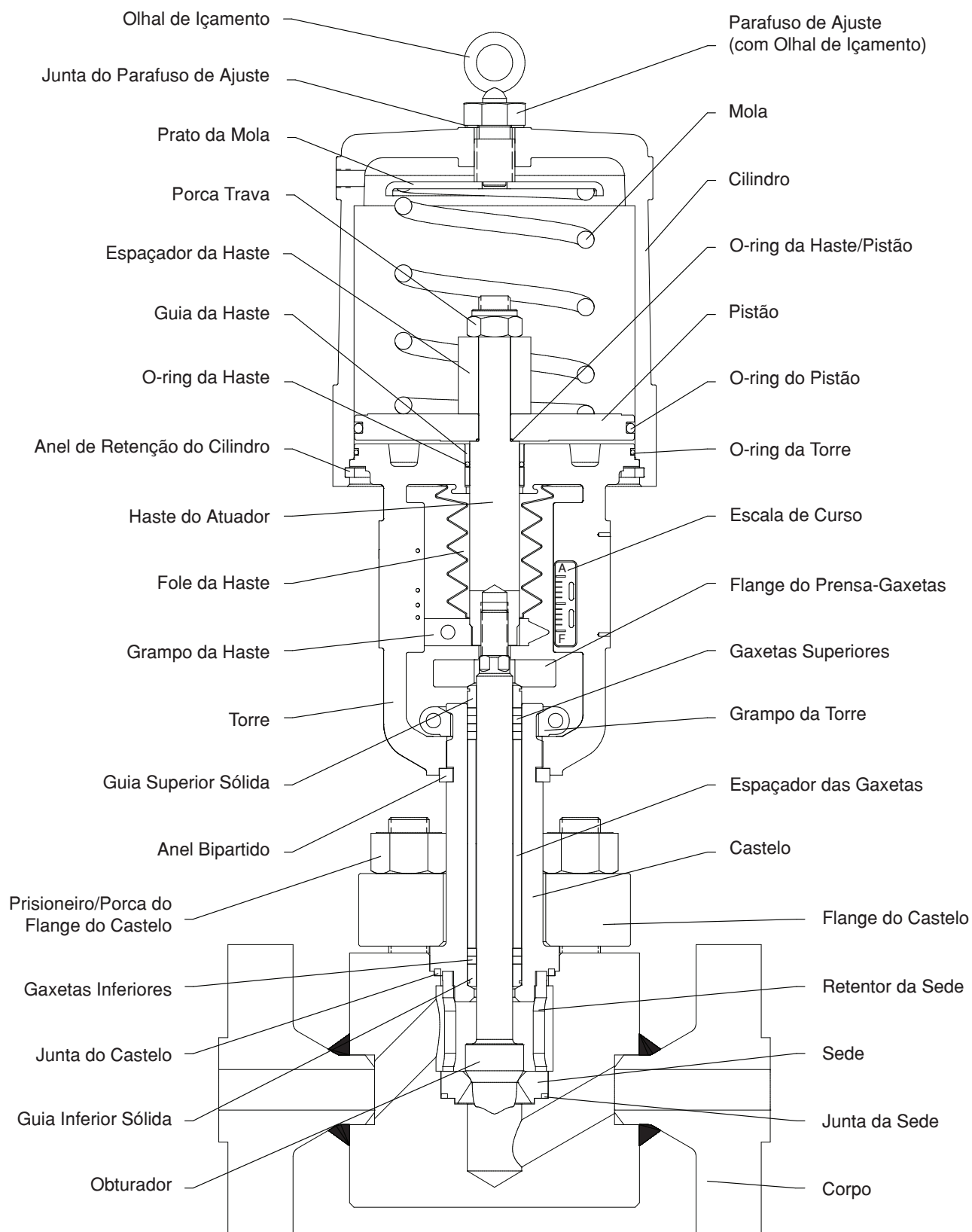
Figura 2 - Válvula de controle GL̄
