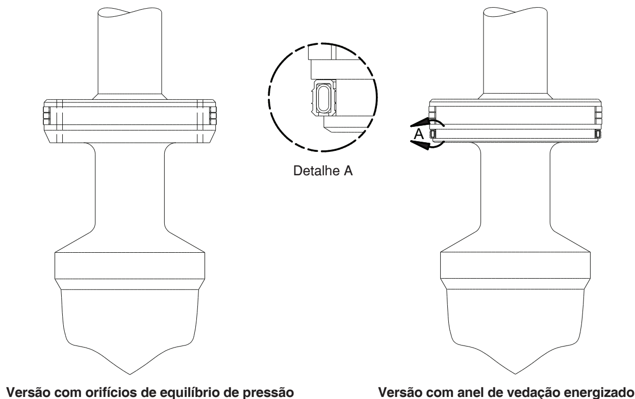
Figura 2 - Mecanismos de Equilíbrio de Pressão dos Obturadores
