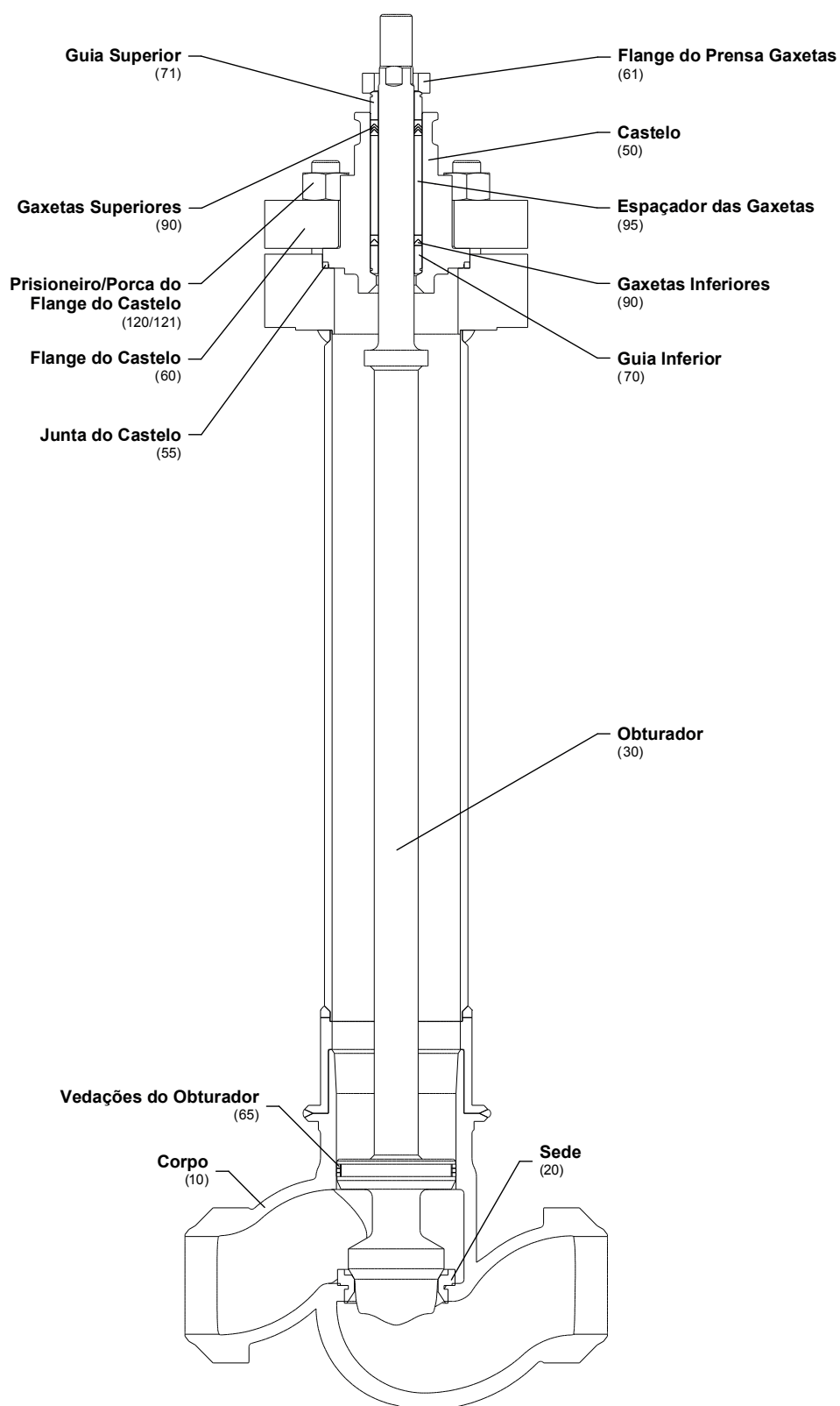
Figura 3 – Válvula de Controle GLc (Subconjunto do Corpo)
