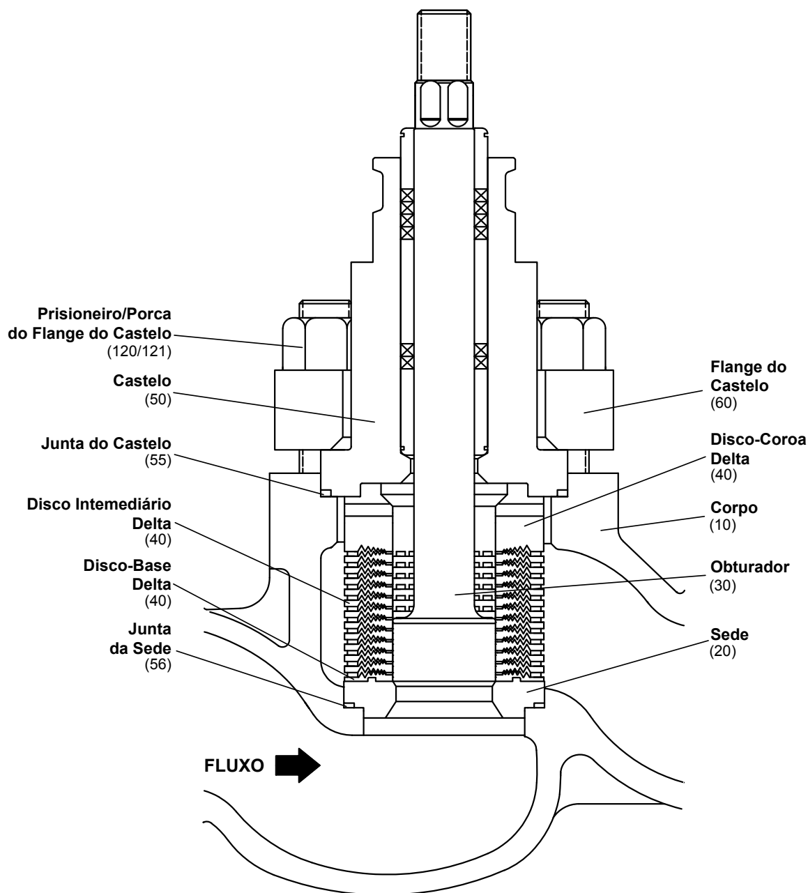
Figura 1 - Válvula com Internos do Tipo Delta Não-Balanceados
