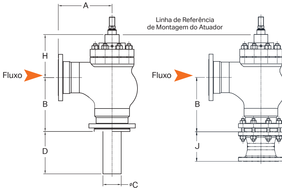
Dimensões (1)(2)
